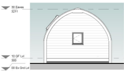
End Elevation 1 : 50
