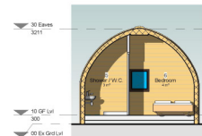
Section A - A 1 : 50
